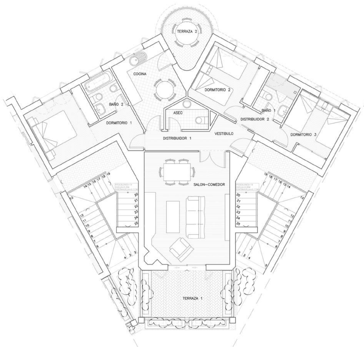
PLANTA PRIMERA. DISTRIBUCION Y MOBILIARIO (viviendas n° : 19)
