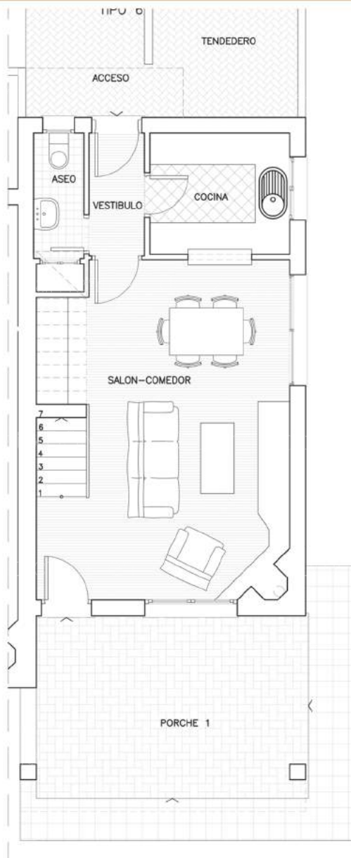
TIPO 6B PLANTA BAJA (viviendas n° : 41)
