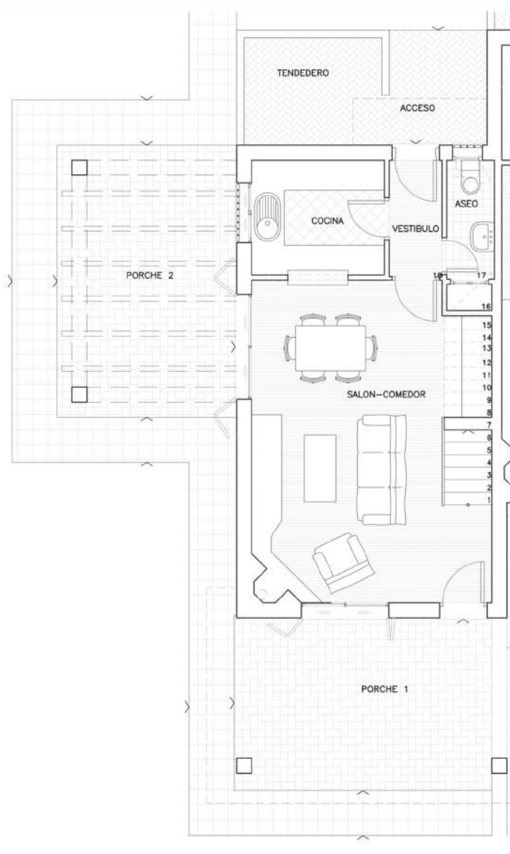
TIPO 6A PLANTA BAJA (viviendas n° : 1)
