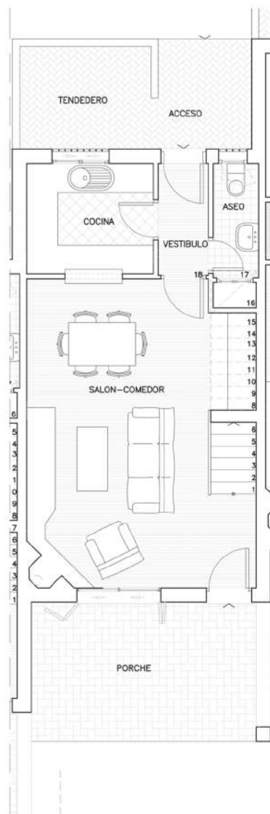
TIPO 5 PLANTA BAJA (viviendas n° : 2-4-5-6-8-9-10-12-30-32-33-34-36-37-38-40)
