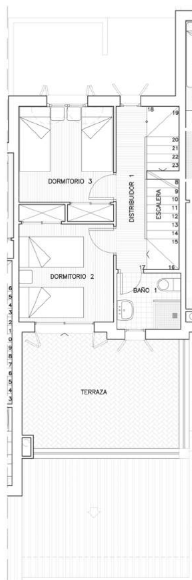
TIPO 4 PLANTA PRIMERA
