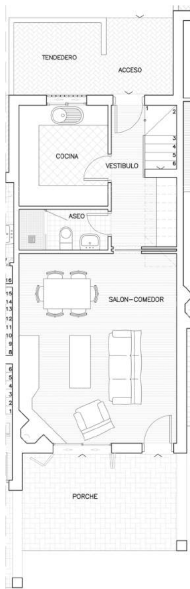
TIPO 4 PLANTA BAJA (viviendas n° : 3-7-11-31-35-39)
