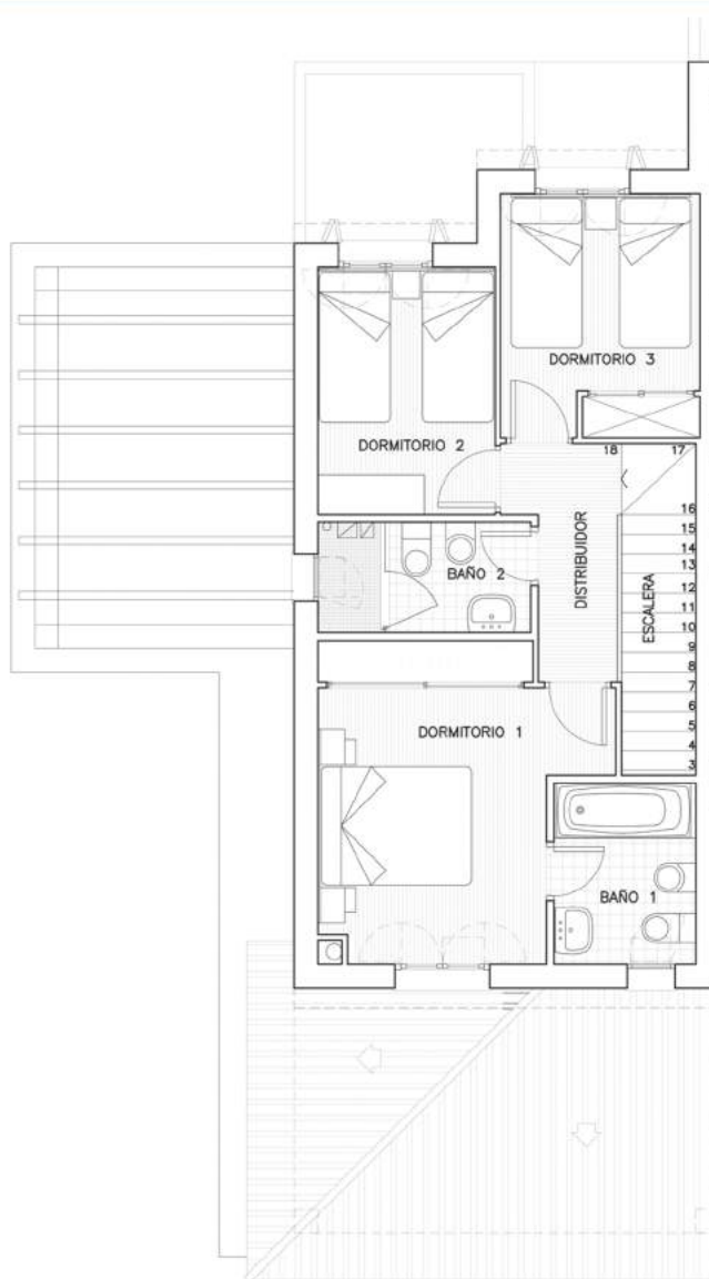
TIPO 6A PLANTA PRIMERA
