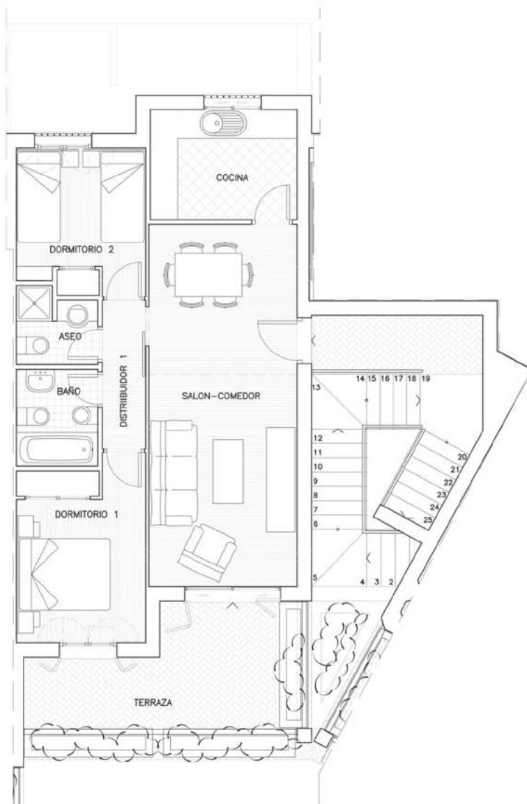
PLANTA PRIMERA DISTRIBUCION Y MOBILIARIO viviendas n° (18-24)
